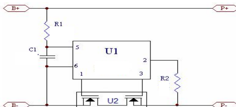
应用原理图
